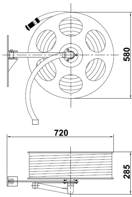
Medidas em (mm)
